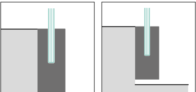
MONTAGGIO LATERALE
